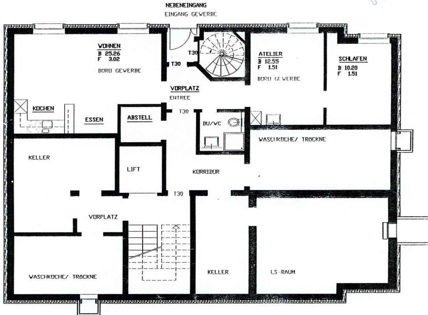
2. UNTERGESCHOSS
